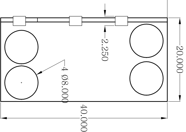
FRONT VIEW VUE AVANT
