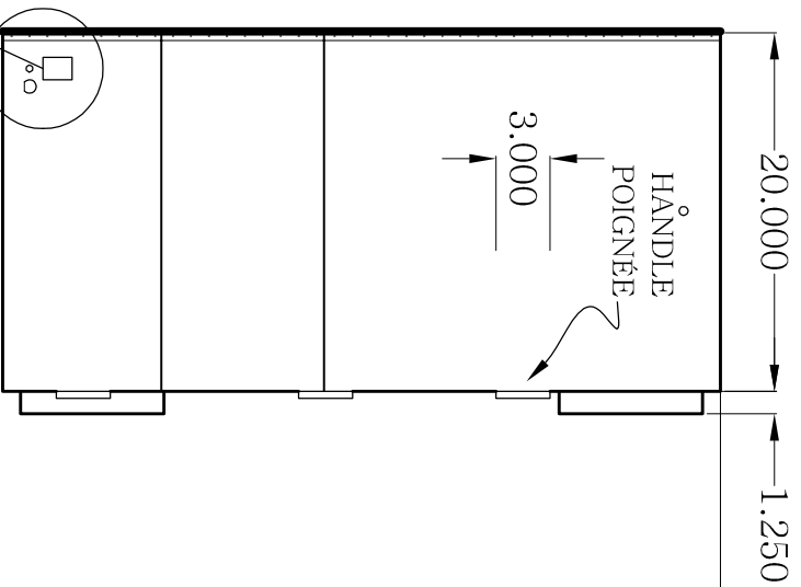
LEFT VIEW VUE GAUCHE
